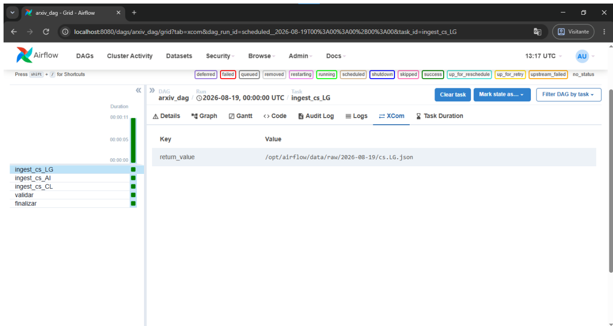
Figura 12. Metadados retornados ao final do DAG executado com sucesso. (autoria própria)
