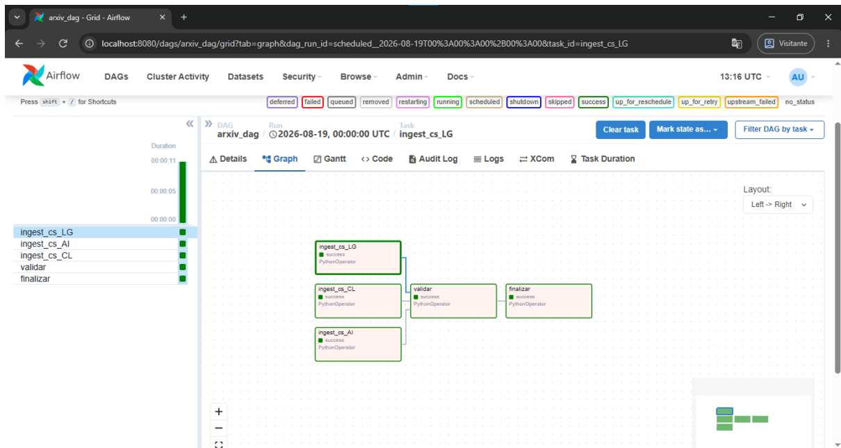
Figura 10. Visualização em grafo do DAG. (autoria própria)
